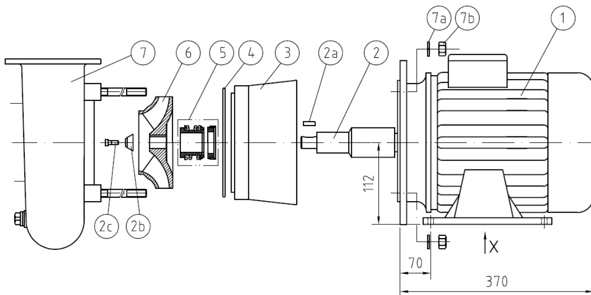
4,0 kW i 5,5 kW 400V typ SB80
